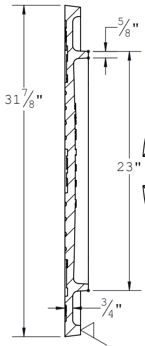
SECTION A-A
