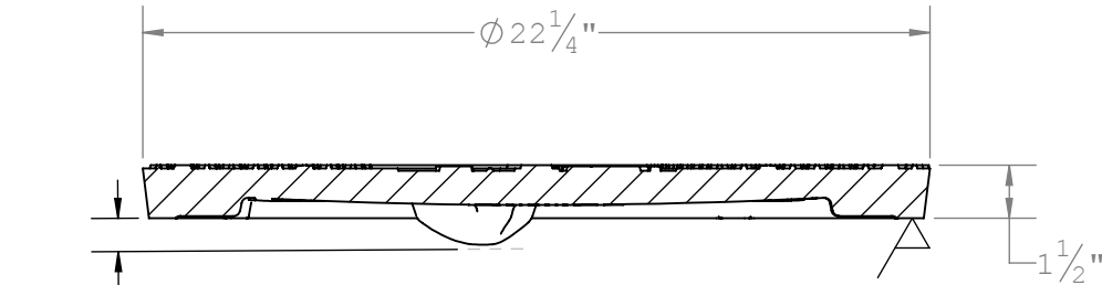
SECTION A-A SCALE 1 : 6
