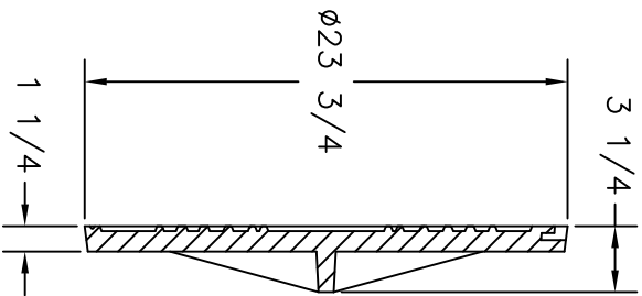
SECTION A-A (Cover)
