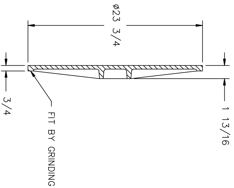
SECTION A-A
