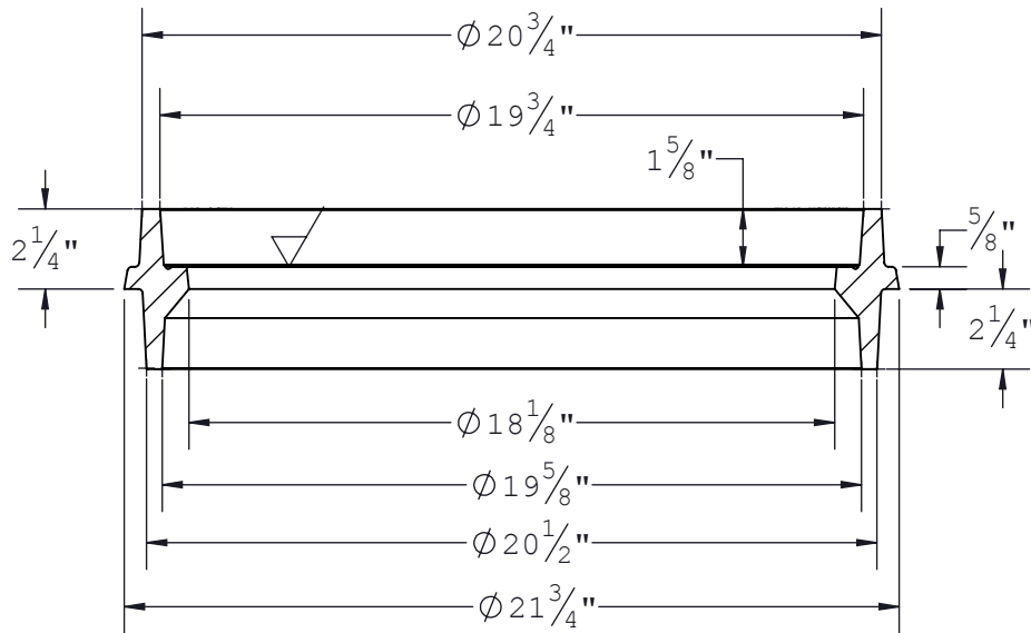
SECTION A-A SCALE 1 : 6
