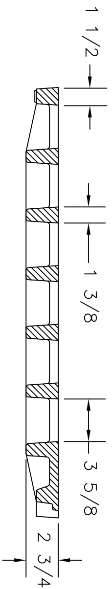
SECTION A-A
