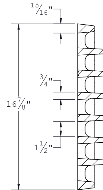
SECTION A-A SCALE 1 : 6
