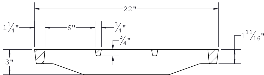
SECTION B-B SCALE 1 : 6
